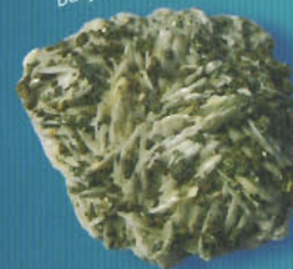
Baryt
